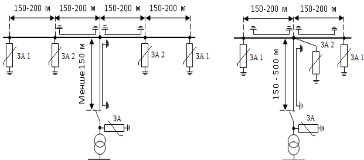
Рисунок 4.2.16 – Схеми спрощеного захисту від грозових перенапруг ПС, приєднаних до ПЛ відгалуженнями.
