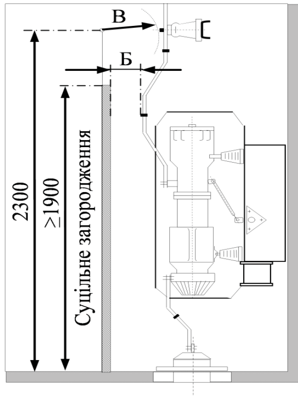
Рисунок 4.2.13 – Найменші відстані між неізолюваними струмовідними частинами в ЗРУ і суцільними загорожами.
