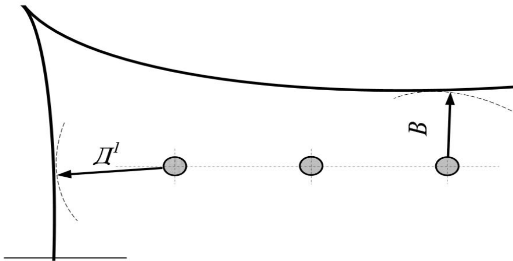
Рисунок 4.2.6 – Найменші відстані між струмовідними частинами різних кіл, розташованими в різних площинах, з обслуговуванням нижнього кола за невимкненого верхнього.
