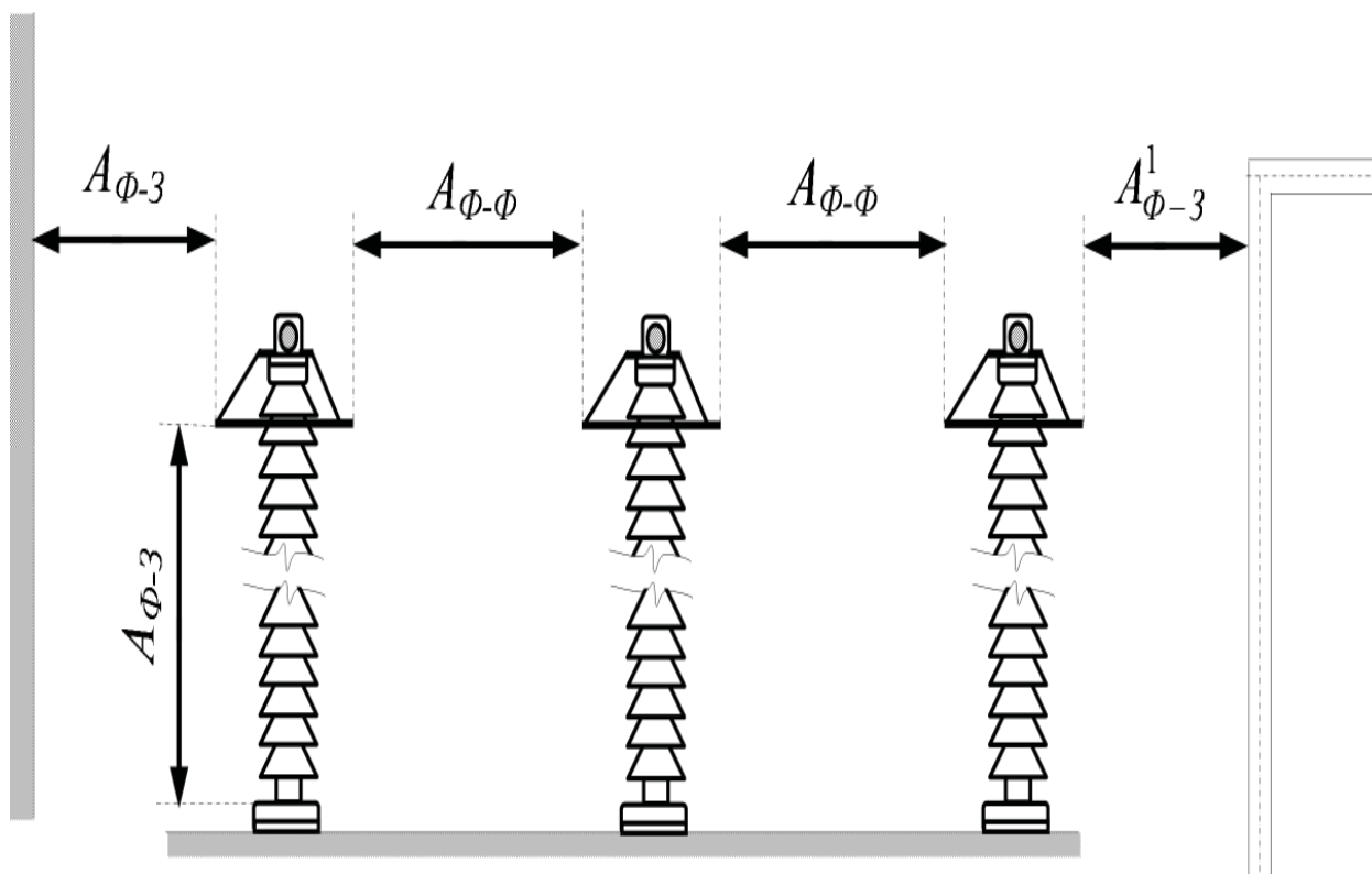
Рисунок 4.2.1 – Найменші відстані в просвіті за жорстких шин між струмовідними і заземленими частинами ( A_{\phi-3} , A_{\phi-3}^I ) та між струмовідними частинами різних фаз ( A_{\phi-\phi} ).
