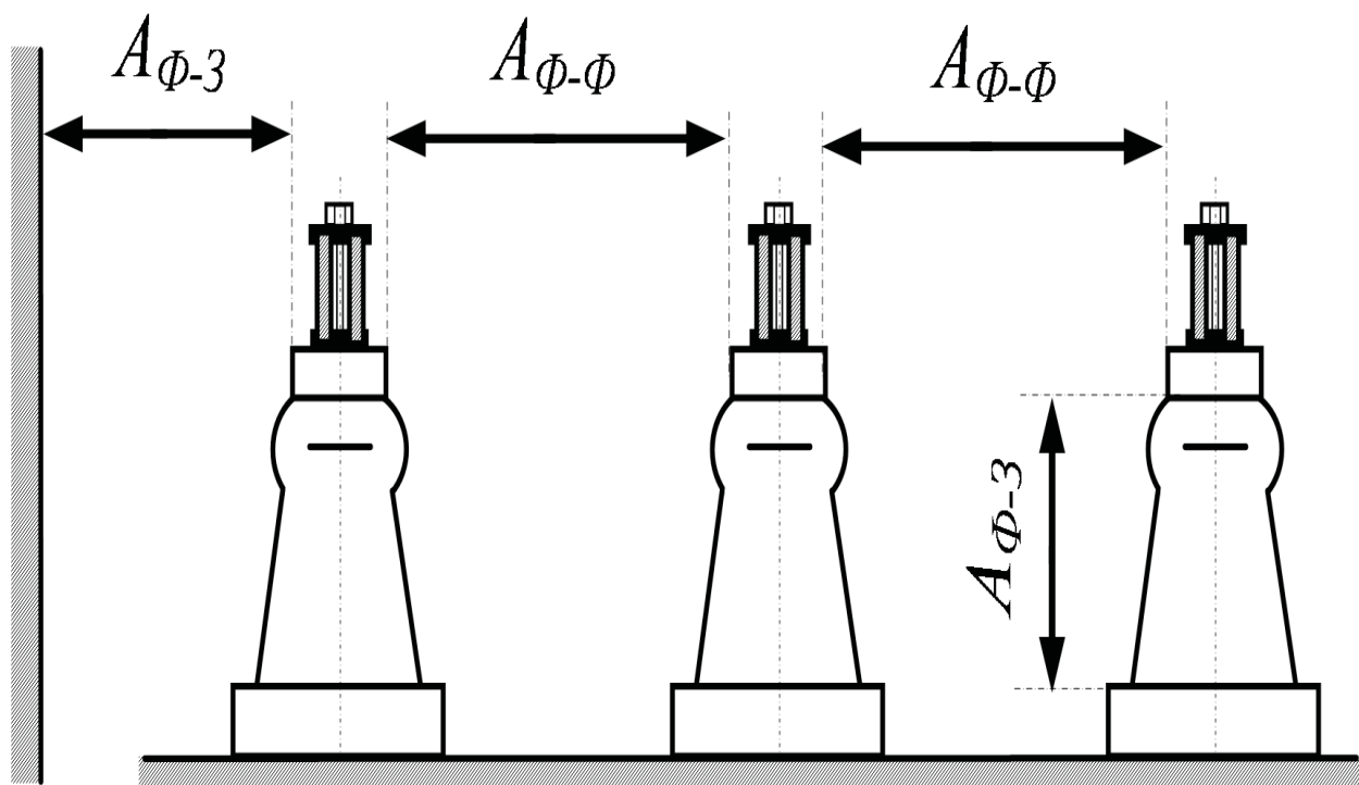
Рисунок 4.2.12 – Найменші відстані в просвіті між неізольованими струмовідними частинами різних фаз у ЗРУ та між ними і заземленими частинами.
